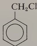
(Chloromethyl)-benzene
