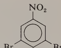
3,5-Dibromonitrobenzene
