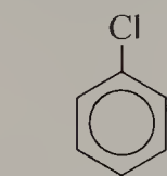
Chlorobenzene
