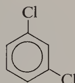
1,3-Dichlorobenzene
