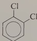
1,2-Dichlorobenzene 1,3-Dichlorobenzene 1,4-Dichlorobenzene
