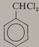
(Dichloromethyl)-benzene
